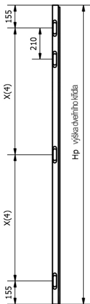
4 závěsy
