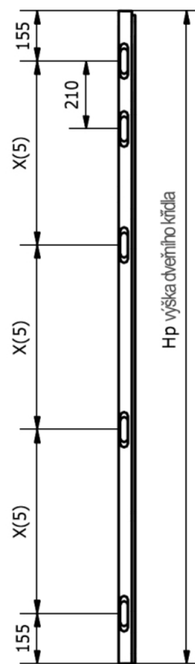
5 závěsů
