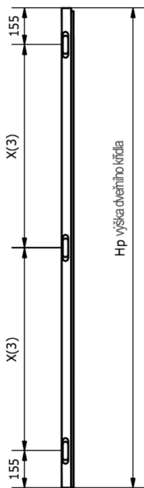
3 závěsy
