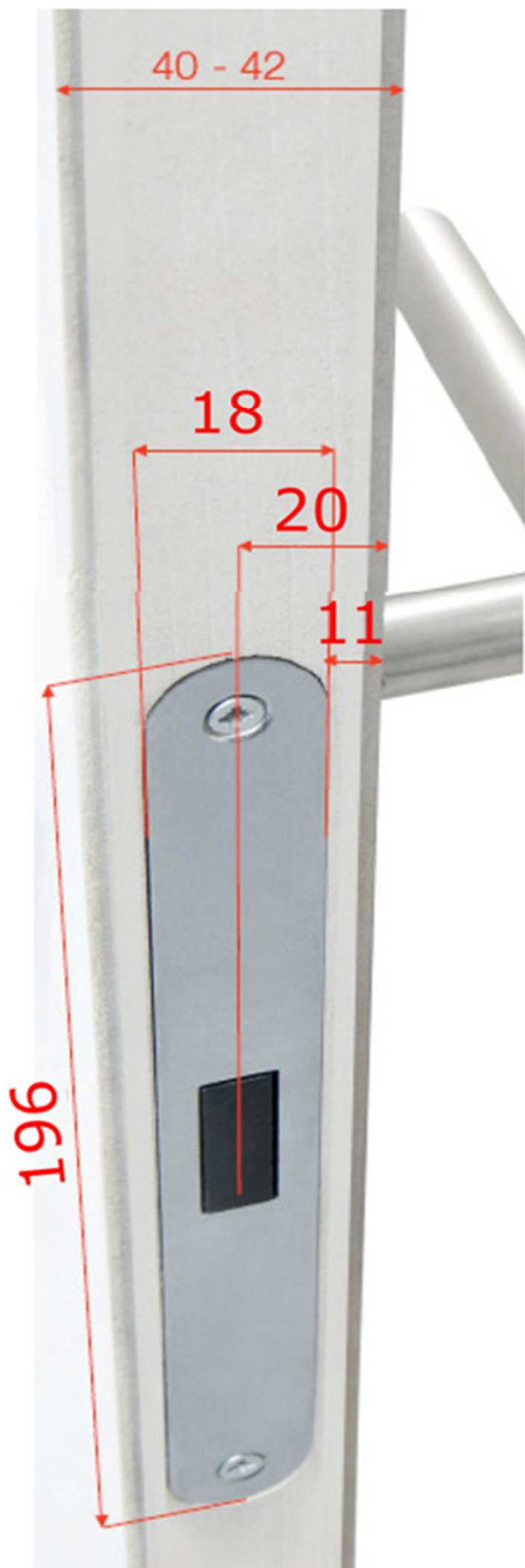
dveře bezfalcové
